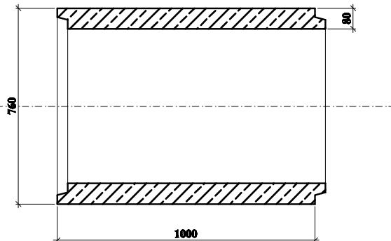
PRZEKRÓJ A-A
